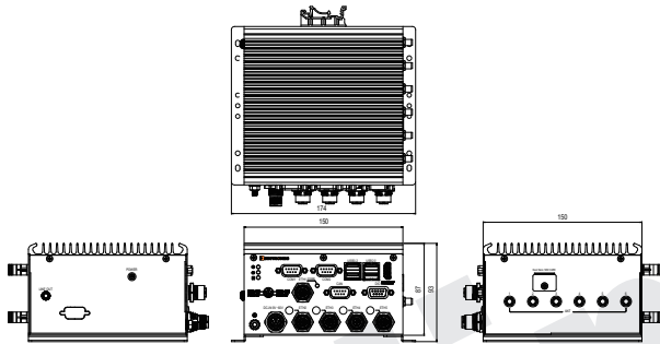
VBOX-3132P-M12X
